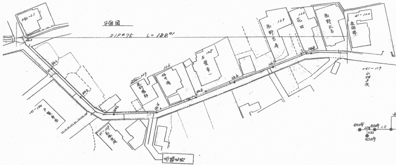
配管図
