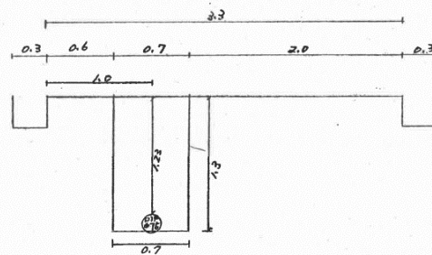
標準断面図
