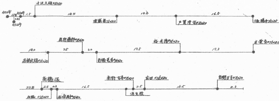
各戸分水栓取付寸法
