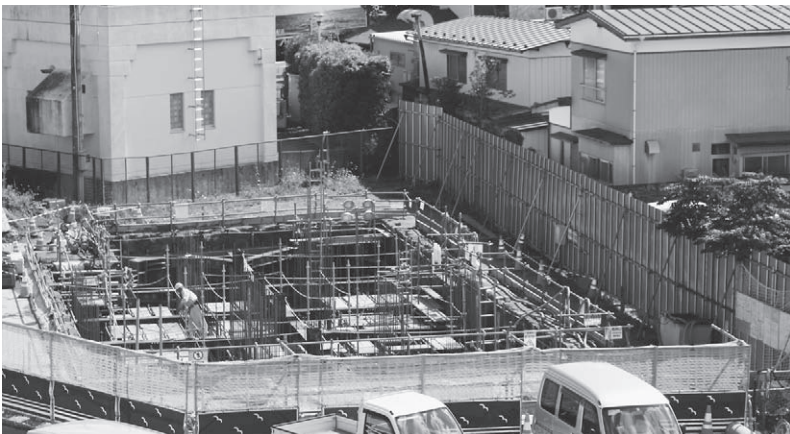
小梨屋雨水ポンプ工事現場
